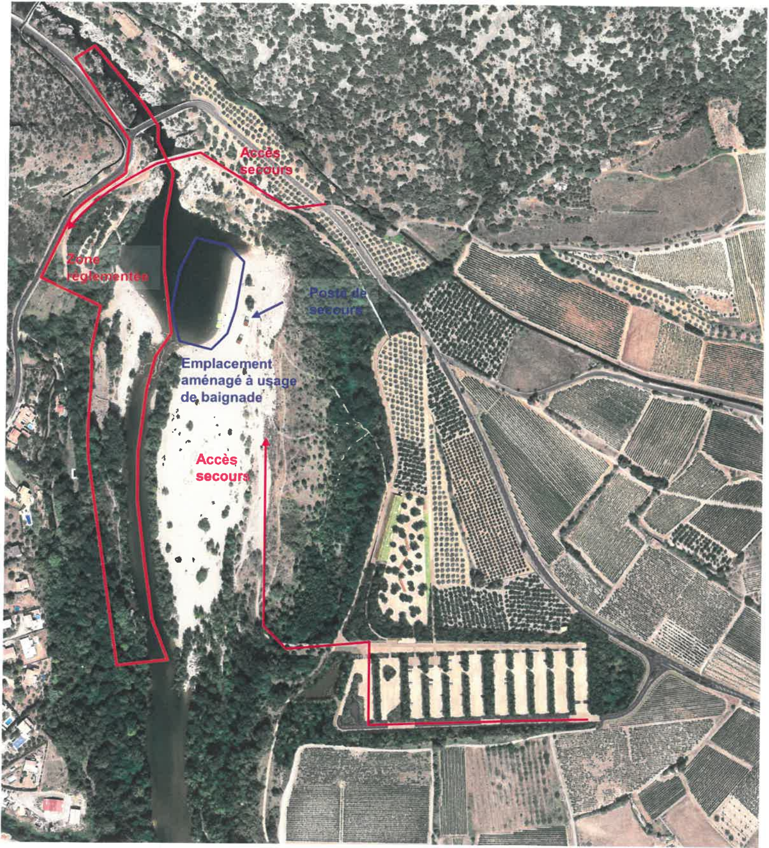
Plan d'implantation – zone réglementée par arrêté municipal n°2022.132 du 01/07/2022 – Site du Pont du Diable
